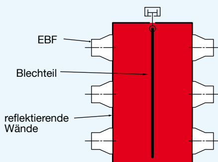
Bild 11: Strahlungstunnel mit mehreren EBF-Systemen
