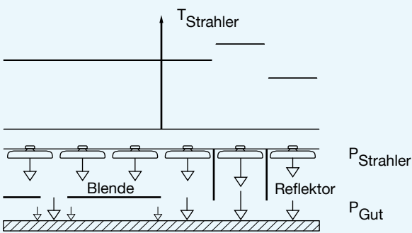
Bild 17: Leistungsanpassung mit Reflektor und Blende
