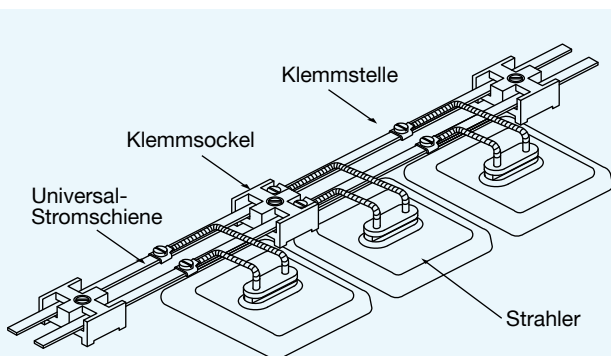
Bild 13: Schienenverdrahtung
