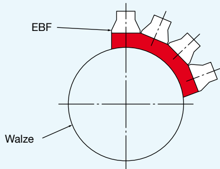
Bild 10: Walzenbeheizung mit dem EBF-System
