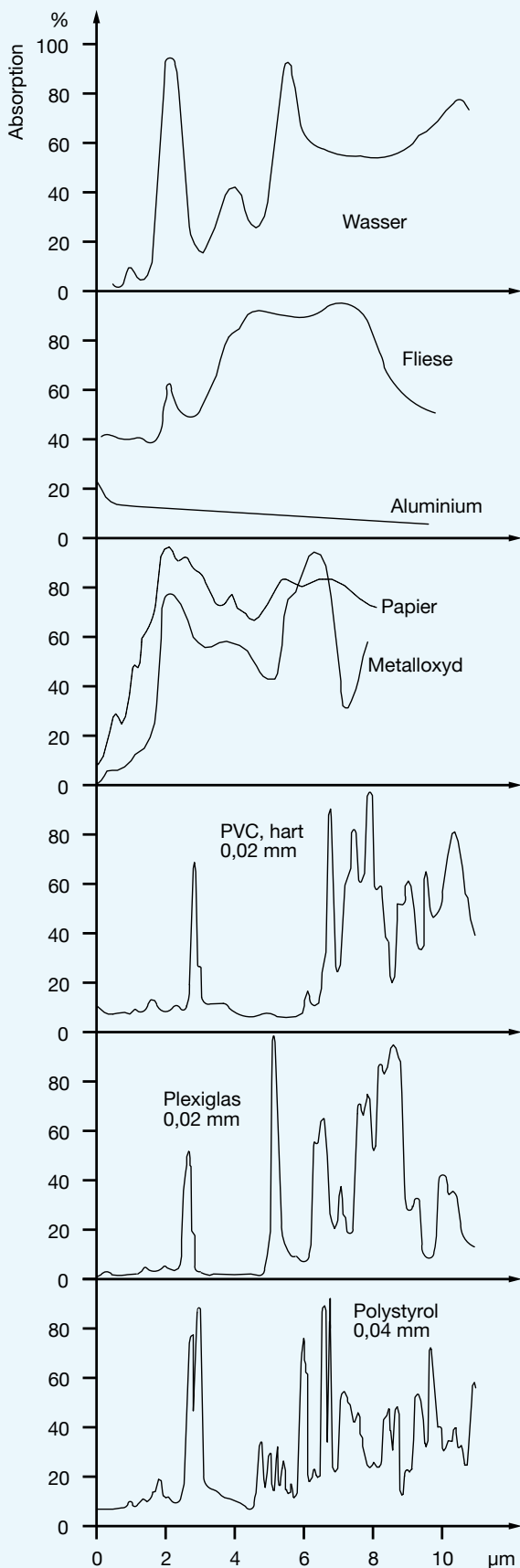
Bild 6: Spektrale Absorption verschiedener Werkstoffe
