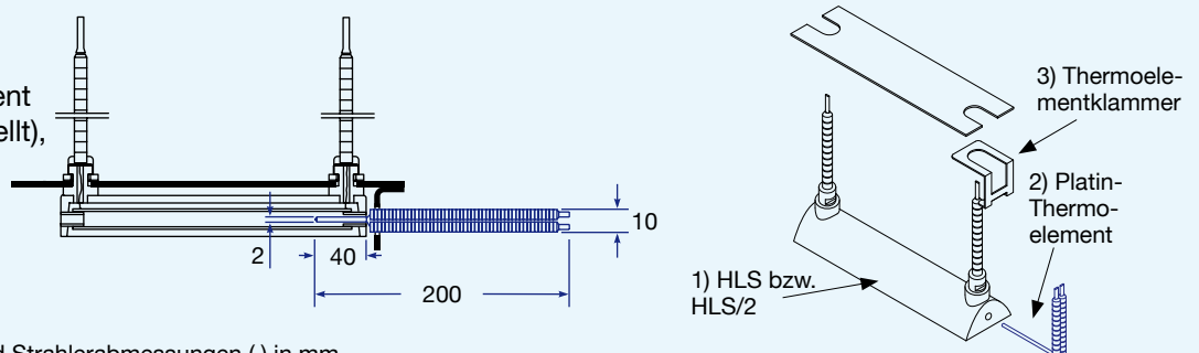
Bild 60: Einbaumaße und Strahlerabmessungen ( ) in mm
