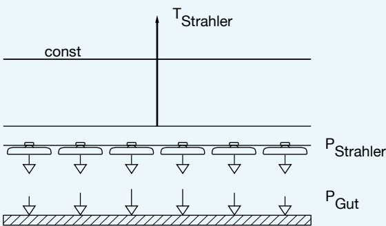
Bild 15: Leistung am Gut bei konstanter Strahlerleistung
